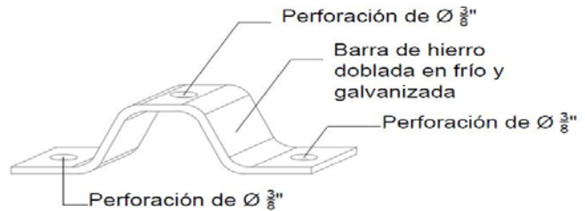
PERSPECTIVA TRAPECIO
